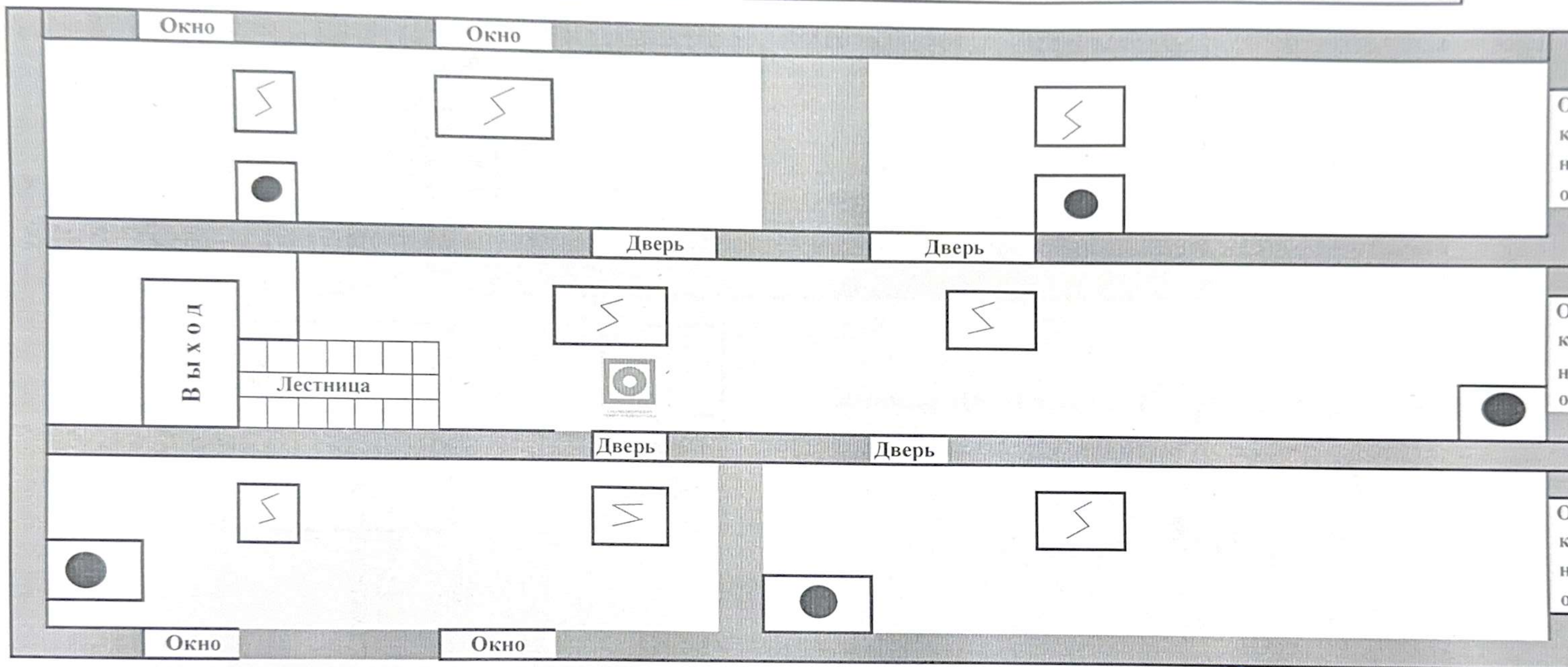
Схема размещения камер видеонаблюдения, датчики дыма, кнопки пожарной безопасности, тревожной кнопки и голосового оповещения. (Второй этаж)
